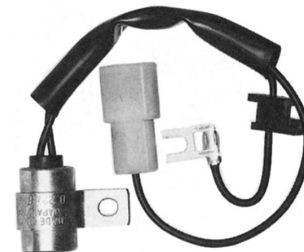
CND-939 MAZDA PART. NO. E303-24-322
