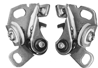
PS-410R, L 22145-60A20 22145-60A21
