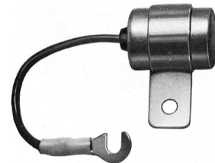
CND-914 MAZDA PART. NO. 0820-24-322 MAZDA CAPELLA R.E. FAMILIA R.E. LUCE A.P. SAVANNA R.E. RX-2, RX-3, R100
